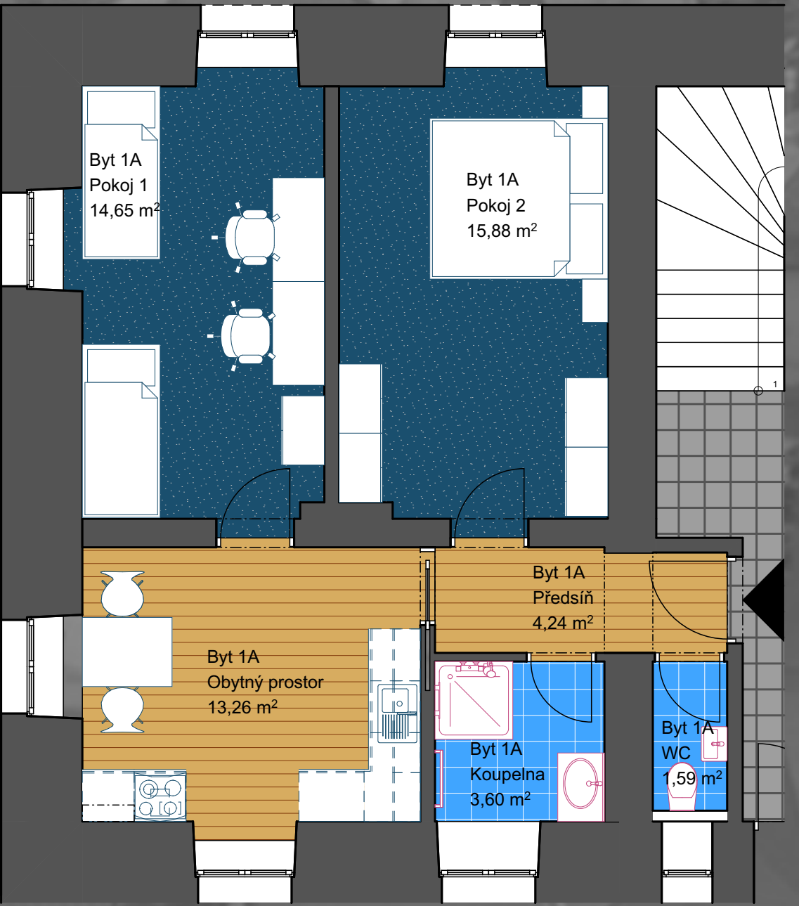
DISPOZIČNÍ ŘEŠENÍ BYTU 1A
